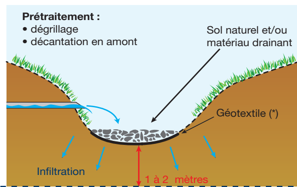
Schéma type (bassin sec)
